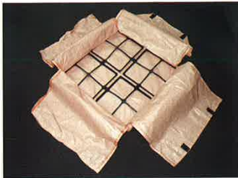
D・BOX-SS90-K 碎石投入量:0.0648 m 3
